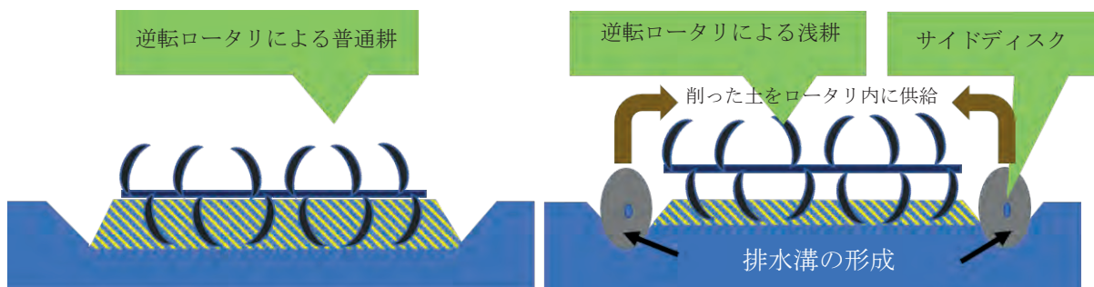
図2 逆転ロータリによる普通耕(左)と浅耕(右)の作業時の畝断面図
