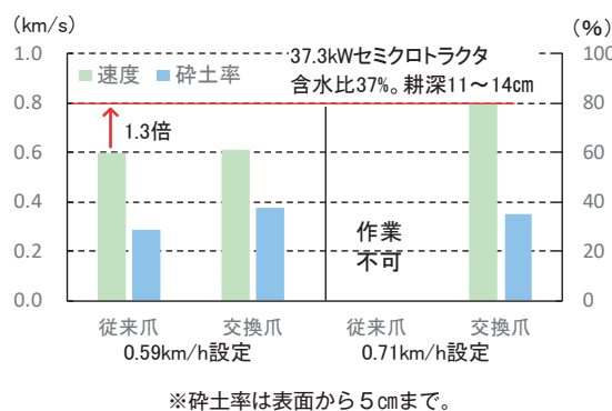
図3 改良爪による速度向上と碎土率
